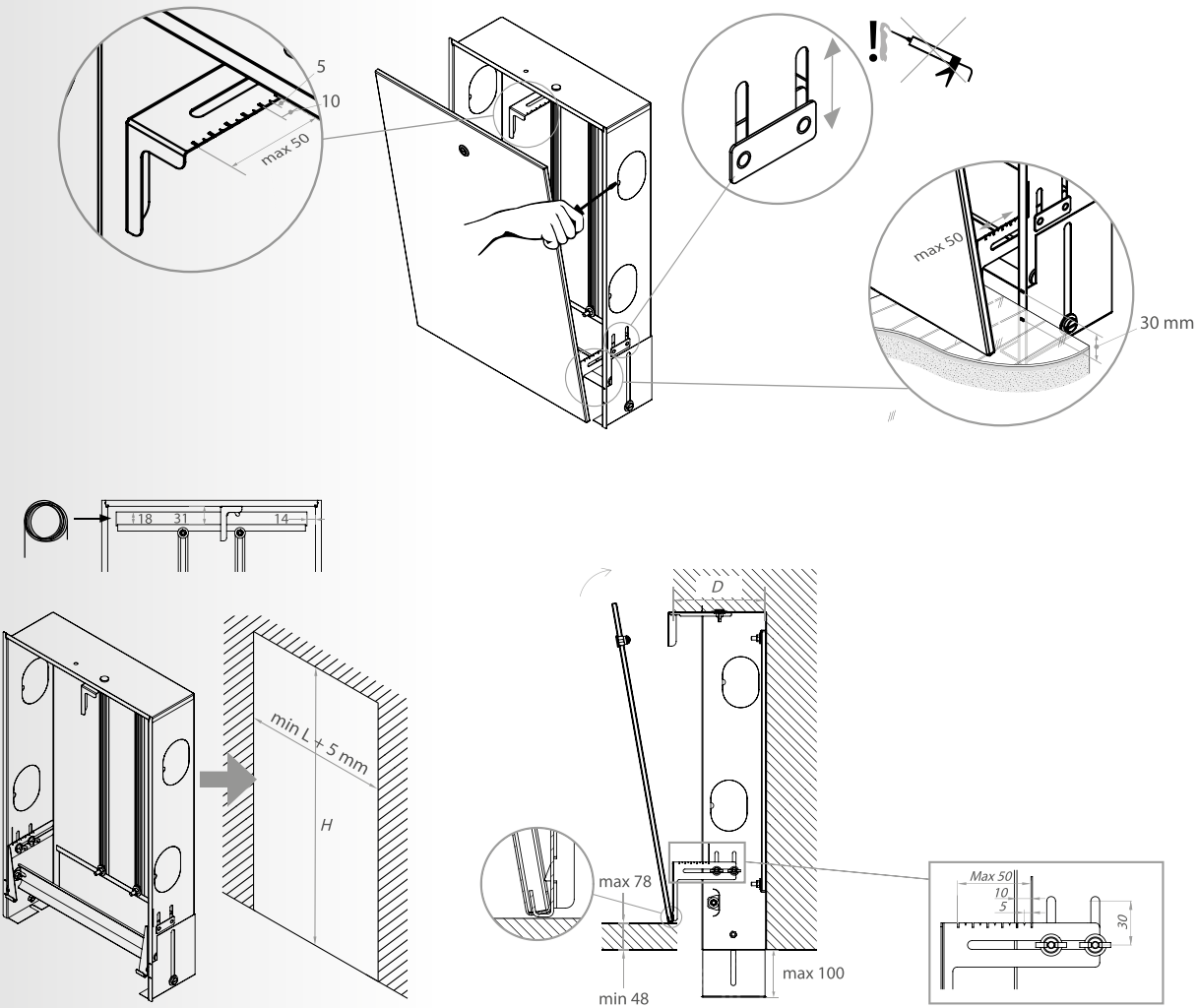
Kappide SPE S paigaldus
