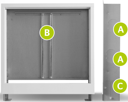
A Külgmised väljalõiked B Paigaldusjuhikud C Kinnitus automaatika jaoks
