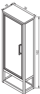
WYMIARY (MM) 360 X 180 X 1020 DIMENSIONS (MM) MATERIAL MATERIAL RAMA ALUMINIOWA, SZKŁO HARTOWANE ALUMINIUM FRAME, TEMPERED GLASS EAN EAN 5900378358176 COLOUR KOLOR CZARNY BLACK
