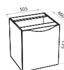
SZAFKA CABINET MODUŁ 20 MODULE
