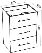
UMYWALKA WASH BASIN KOLORADO 60
