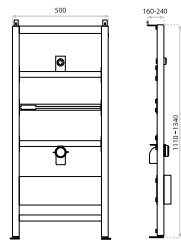
STELAZ DO PODTYNKOWEGO MONTAŻU PISUARU FRAME FOR CONCEALED INSTALLATION OF URINAL LAV 600 DIMENSIONS (MM) WYMIARY (MM) 1110-1340 x 500 x 160-240 EAN EAN 5908211494876
