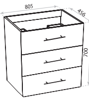
UMYWALKA WASH BASIN KOLORADO 80
