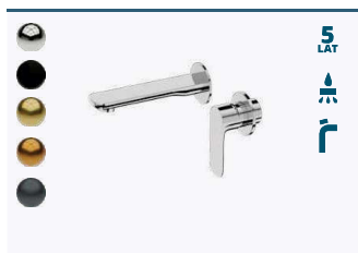
BATERIA UMYWALKOWA PODTYNKOWA CONCEALED WALL FAUCET SPARK MATERIAL MATERIAL MOSIĄDZ BRASS ESCUTCHEON SIZE ROZMIAR ROZETY SR-60 114-110 SPOUT REACH FROM TILES ZASIĘG WYLEWKI OD PŁYTEK 177
