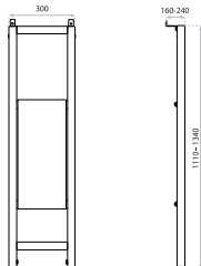
STELAZ DO PODTYNKOWEGO MONTAŻU UCHWYTU DLA NIEPEŁNOSPRAWNYCH FRAME FOR FLUSH MOUNTING OF THE HANDLE FOR THE DISABLED LAV 700 DIMENSIONS (MM) WYMIARY (MM) 1110-1340 x 300 x 160-240 EAN EAN 5908211494883
