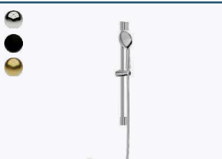
ZESTAW PRYSZNICOWY Z DRAŻKIEM ORION MATERIAL MATERIAL ABS ABS SHOWER HOSE, LENGTH WĄZ PRYSZNICOWY, DŁUGOŚĆ 1500 SHOWER HANDLE / NUMBER OF FUNCTIONS RĄCZKA PRYSZNICOWA / ILOŚĆ FUNKCJI 5 FUNKCJI / 5 FUNCTIONS
