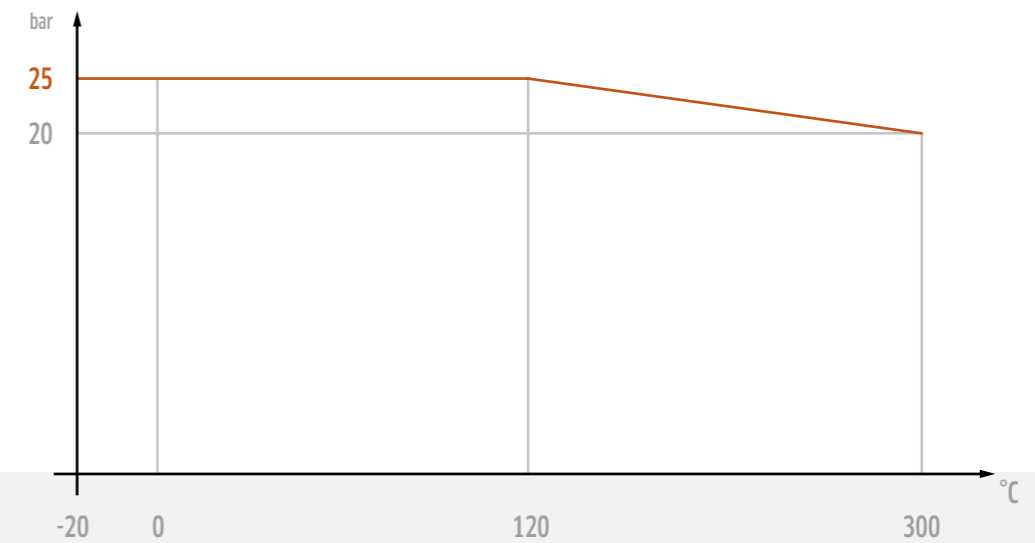
Diagramm: Druck/Temperatur
