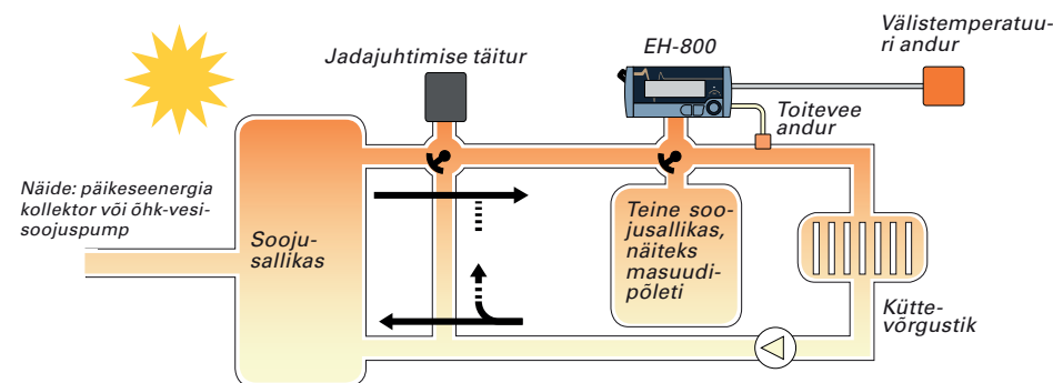
Jadajuhtimise põhidiagramm
